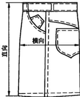
图 4 短裙水洗前后测量部位示例
